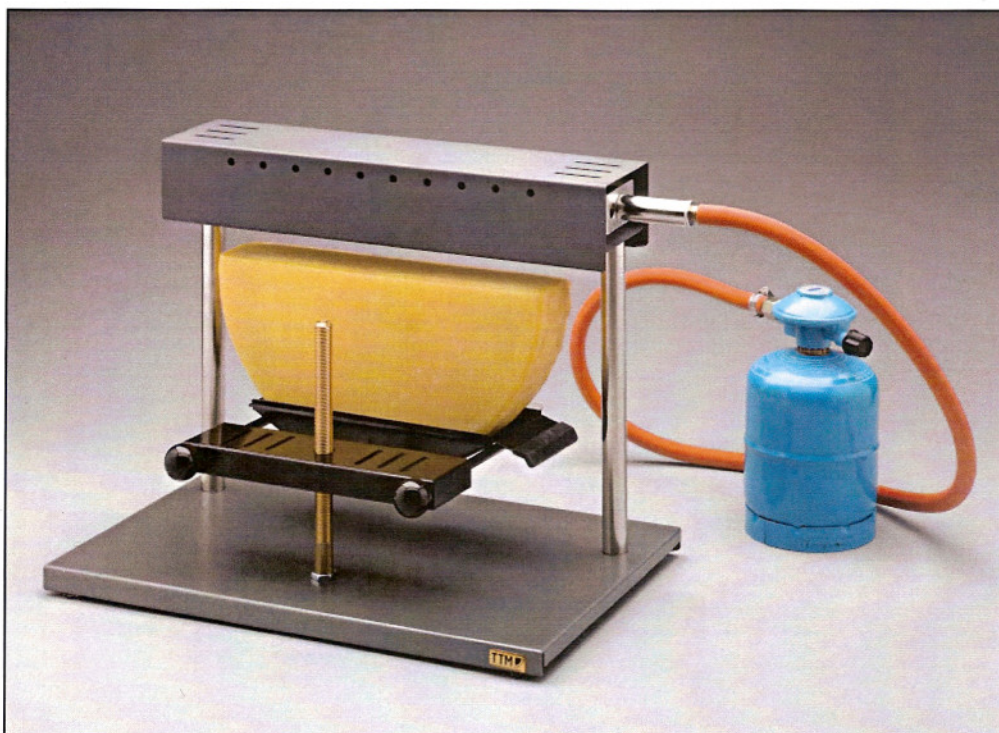
Art. 100.028, Racletteofen EASY-GAZ für einen halben Raclettekäse
